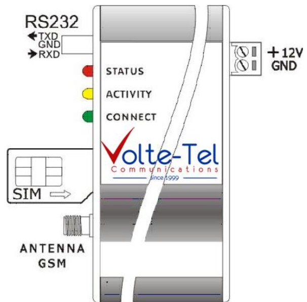
Σχήμα 1: Συνδέσεις του FCT-5
